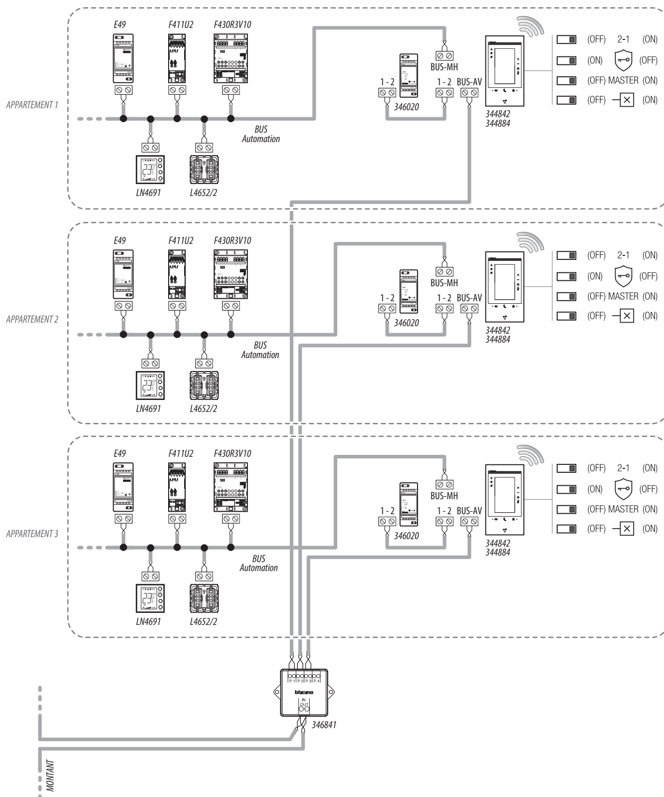
SCHÉMA 3 - EXEMPLE D'INSTALLATION MULTI-FAMILLE AVEC ALIMENTATEUR ET AVEC BUS AUTOMATION
