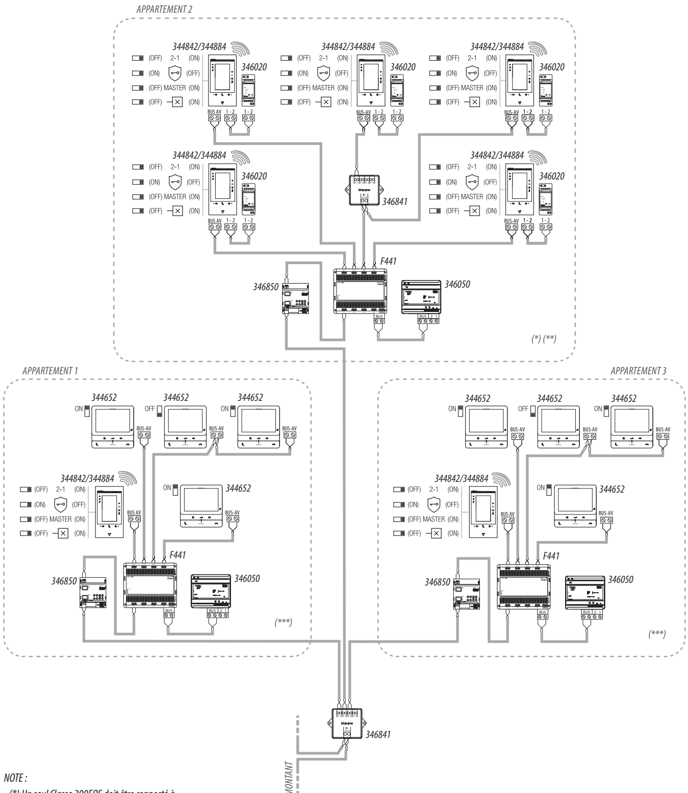
SCHÉMA 5 - EXEMPLE D'INSTALLATION MULTI-FAMILLE AVEC INTERFACE D'APARTEMENT 346850
