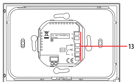
Versión de empotrar
