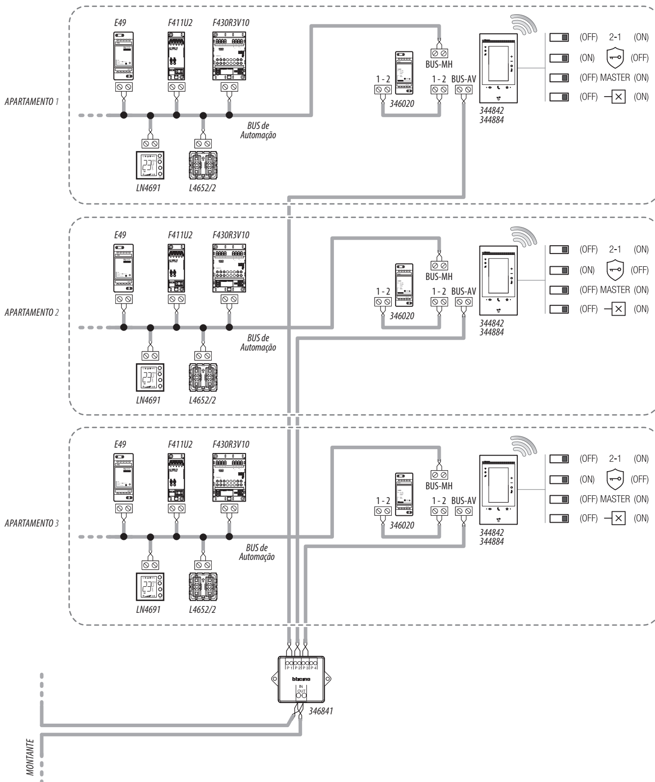
DIAGRAMA 3 - EXEMPLO DE UM SISTEMA MULTI-FAMILIAR COM ALIMENTADOR E COM BUS DE AUTOMAÇÃO
