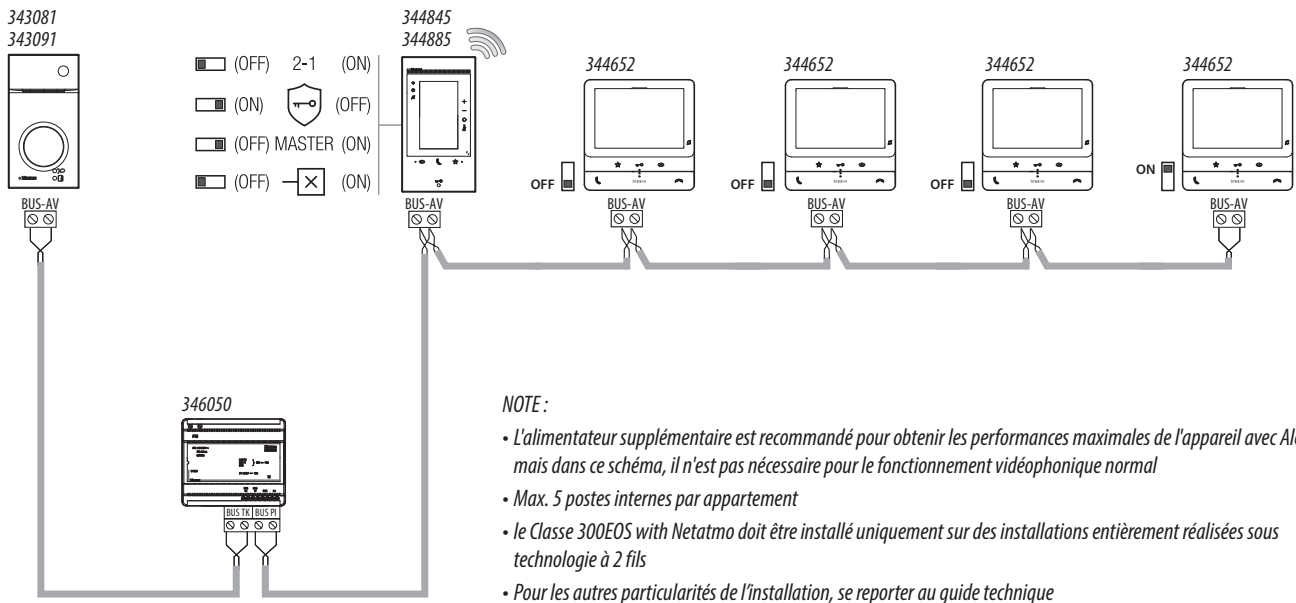
SCHÉMA 6 - EXEMPLE D'INSTALLATION MONO-FAMILIALE
