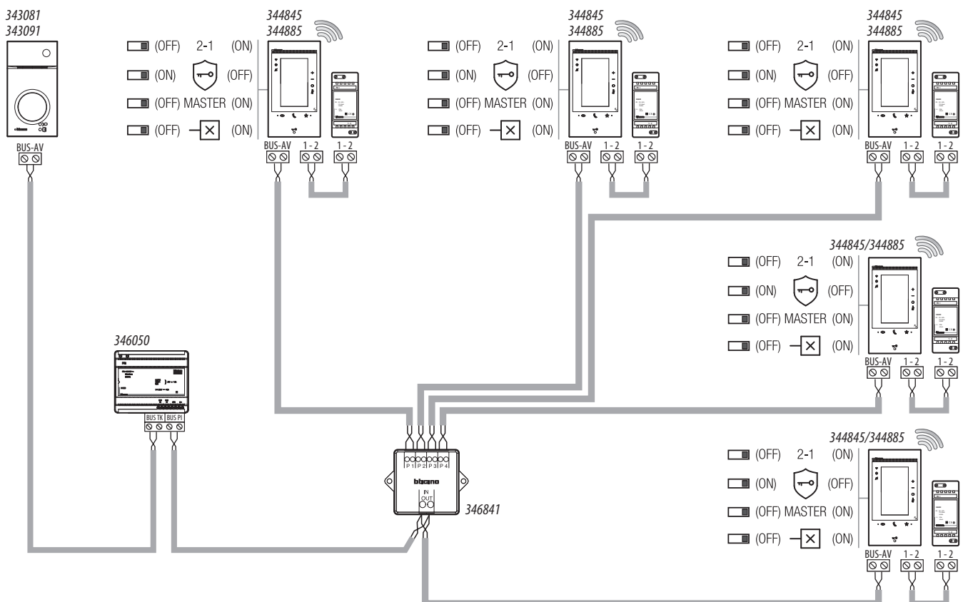
SCHÉMA 7 - EXEMPLE D'INSTALLATION MONO-FAMILIALE AVEC 5 CLASSE 300EOS WITH NETATMO
