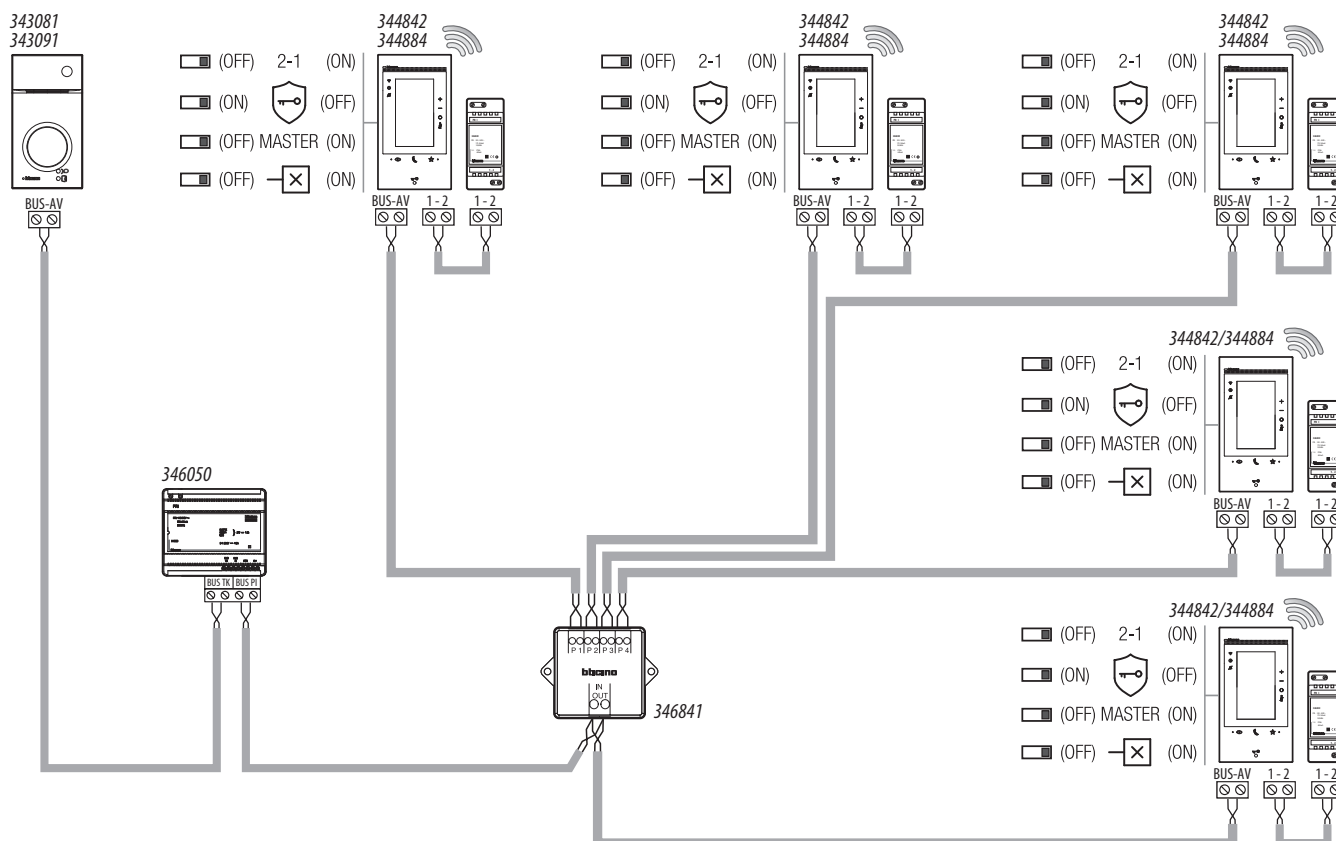
ESQUEMA 7 - EJEMPLO ESQUEMA MONOFAMILIAR CON 5 CLASSE 300EOS WITH NETATMO
