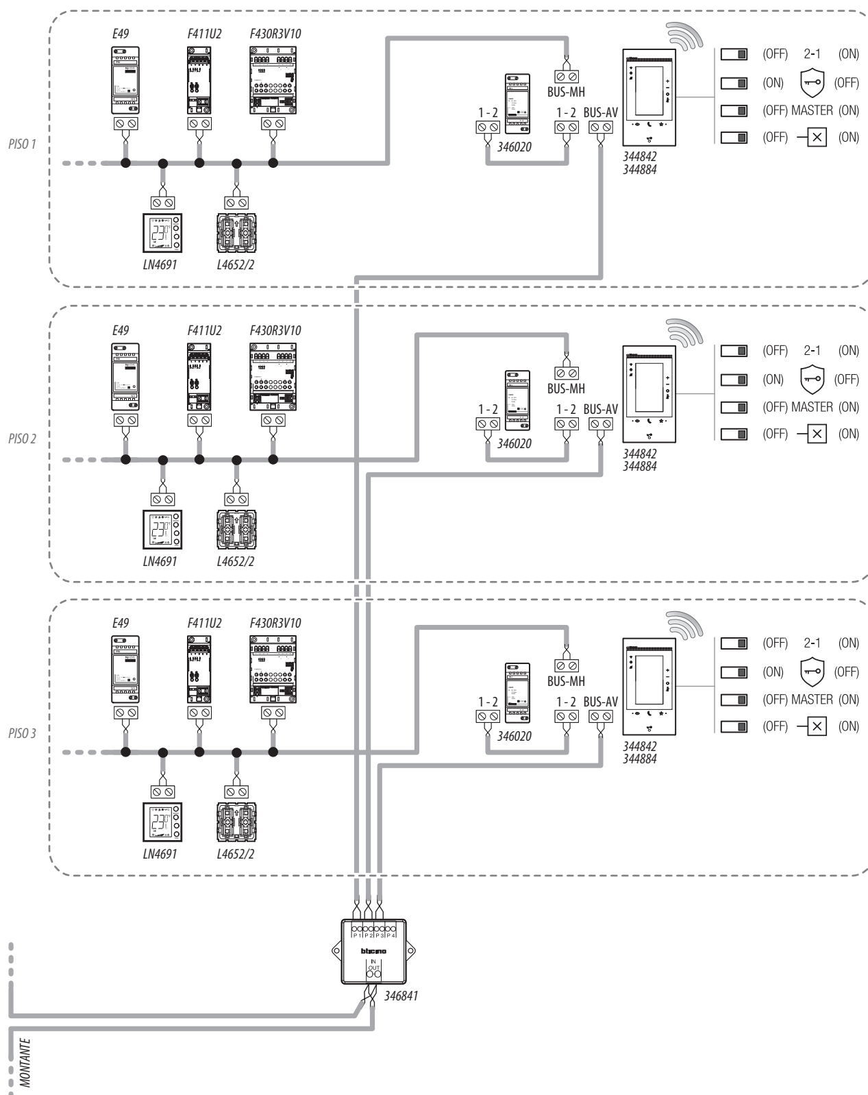
ESQUEMA 3 - EJEMPLO INSTALACIÓN PLURIFAMILIAR CON ALIMENTADOR Y CON BUS AUTOMATISMO
