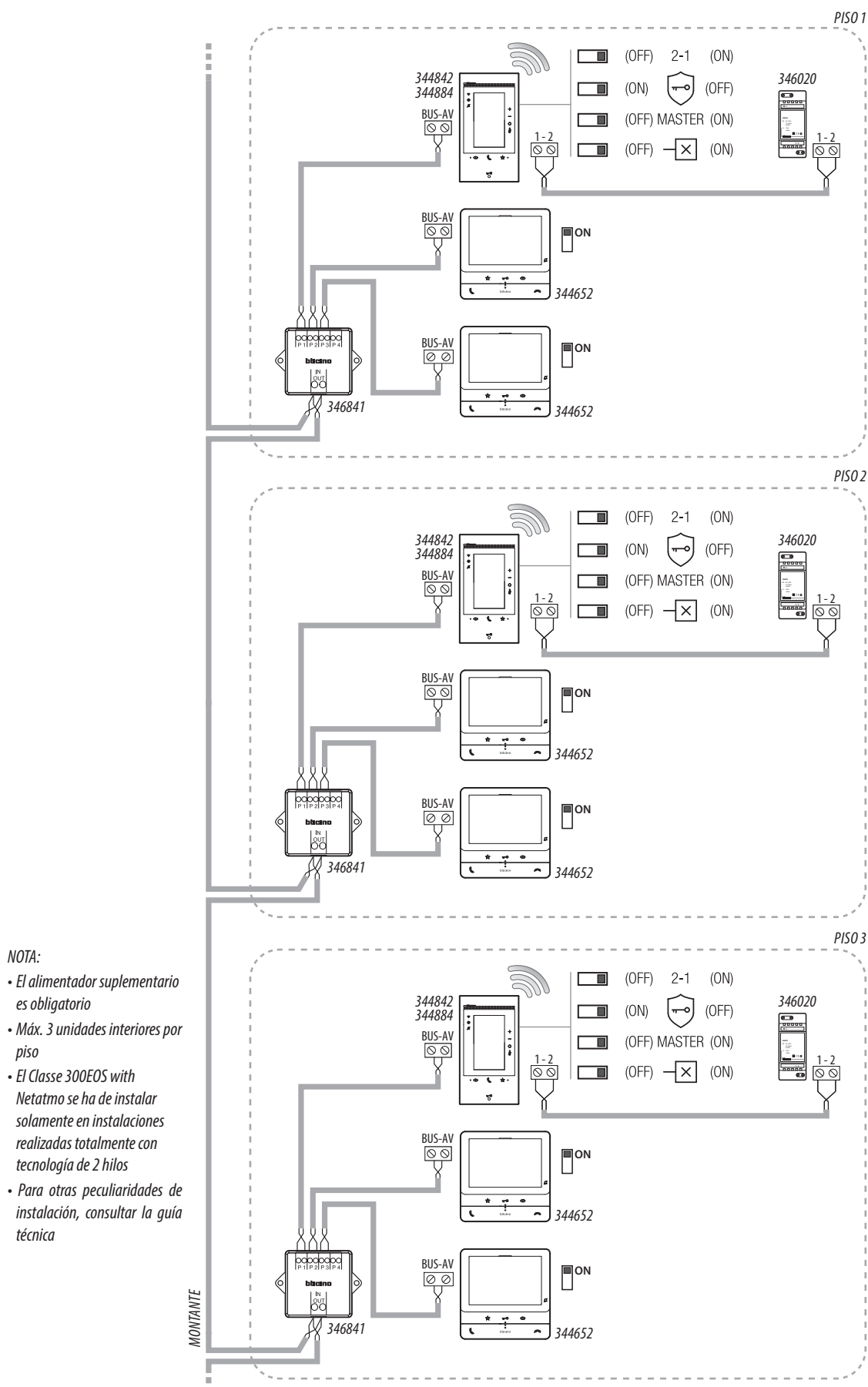
ESQUEMA 4 - EJEMPLO INSTALACIÓN PLURIFAMILIAR CON UNIDADES DE INTERIOR ADICIONALES
