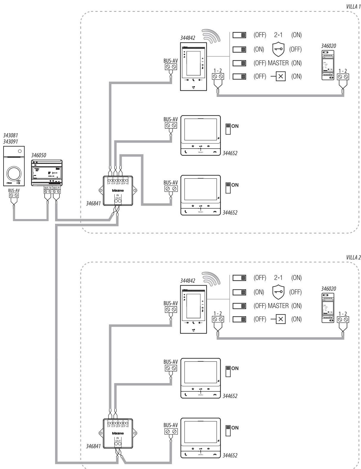
SCHEMA 8 - VOORBEELD VAN EEN TWEEGEZINS INSTALLATIE
