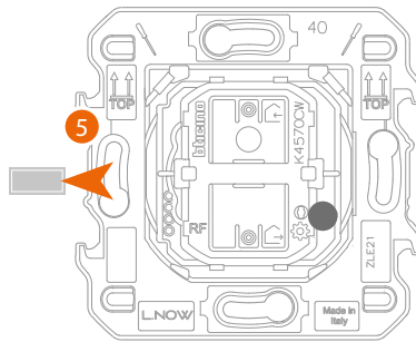
Comandă scenarii Intrare&leșire wireless master
