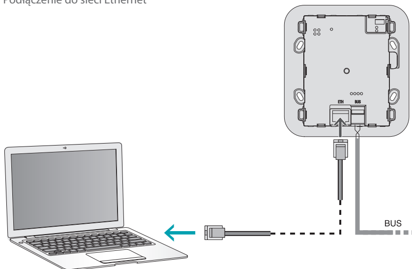
Podłączenie do sieci Ethernet
