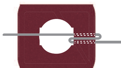
2 Passages de câble 75/5A 2 Cable passages 75/5A
