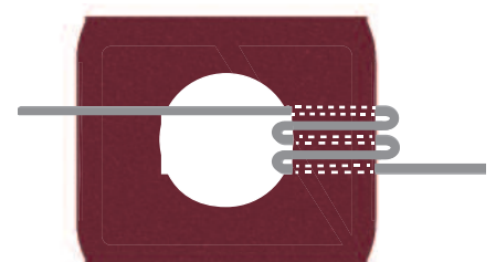
3 Passages de câble 50/5A 3 Cable passages 50/5A
