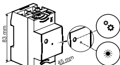
Brama modułowa
