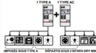
Schéma de câblage à l'intérieur
