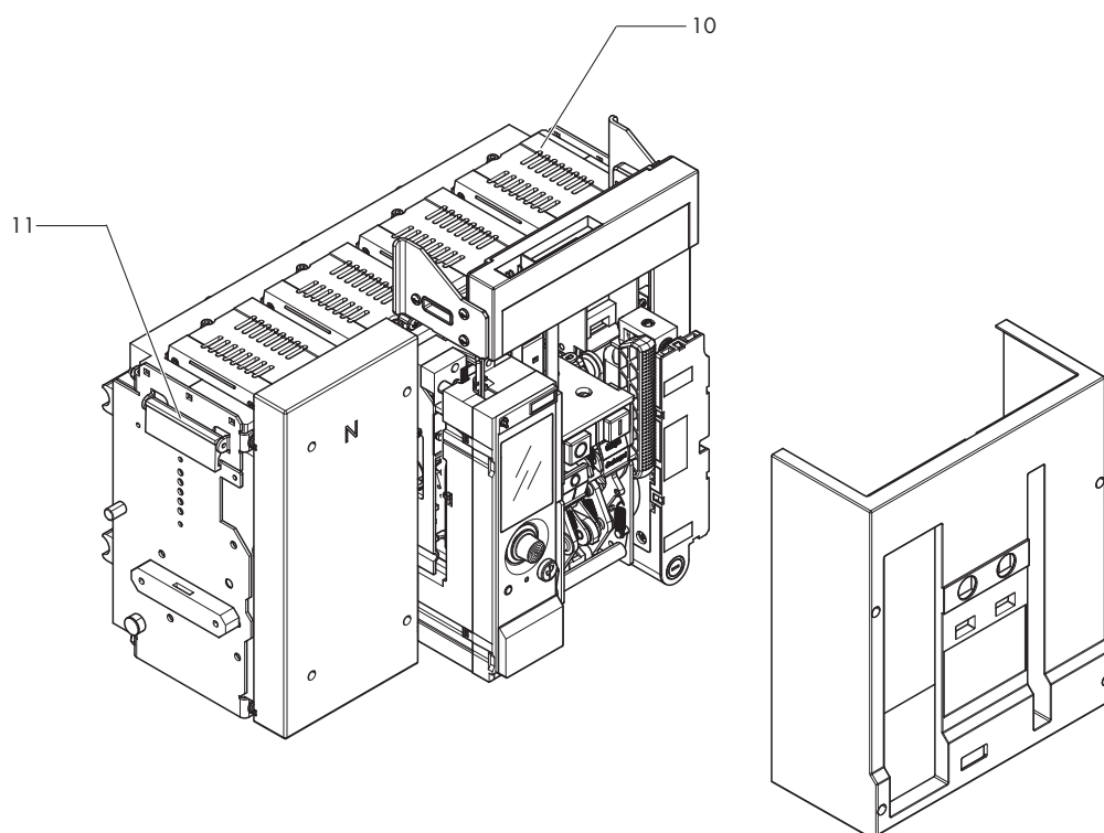
Version partie mobile
