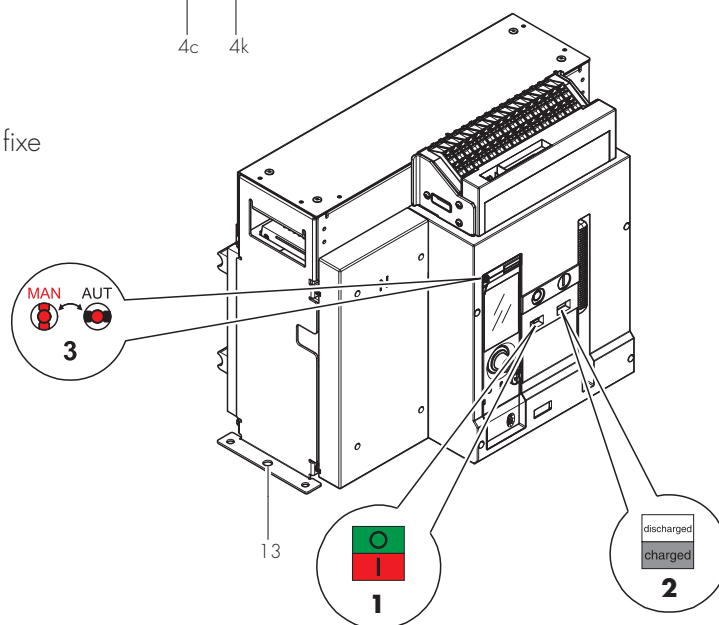
Version débrochable
