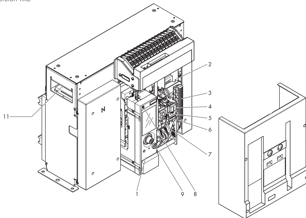
Version partie mobile
