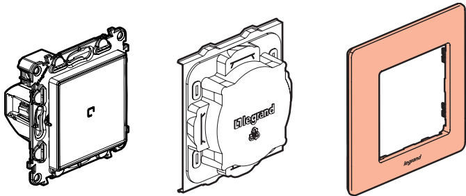
Συνδεδεμένος διακόπτης με ουδέτερο (με δυνατότητα dimmer)
