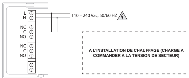
Installation pour chauffage uniquement avec charge à commander à la tension de secteur (ex. électrovanne 230 V)
