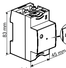
Gateway module
