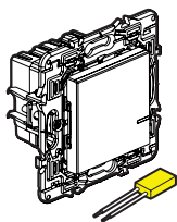
Interrupteur (avec option variateur) connecté + compensateur
