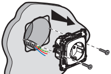
Демонтируйте имеющуюся розетку
