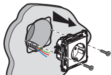
Demontați priză existentă
