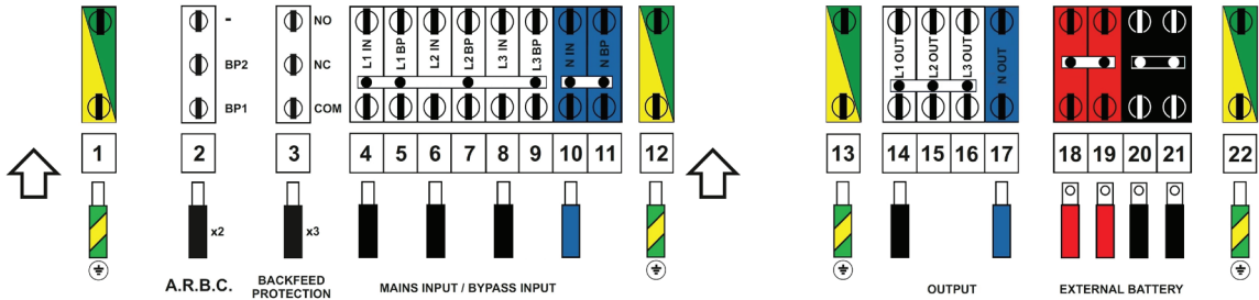
Trimod MCS 30 con linea di ingresso bypass in comune
