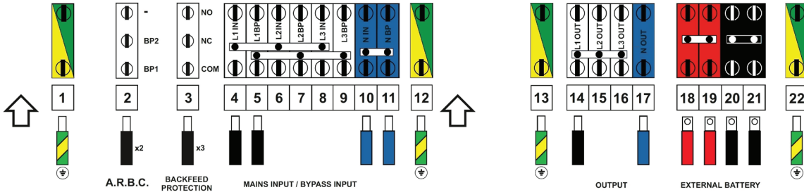
Trimod MCS 30 con linea di ingresso bypass separata
