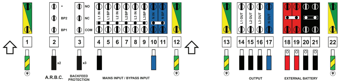
Trimod MCS 30 con linea di ingress bypass in comune
