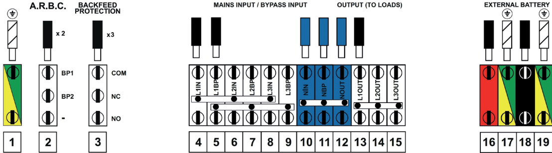
Trimod MCS 10 - 15 - 20 con linea di ingresso bypass separata
