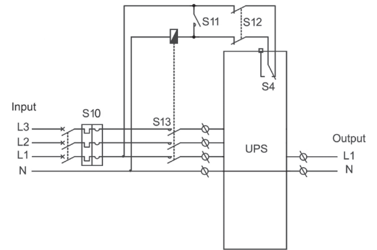
Configurazione Trifase/Monofase
