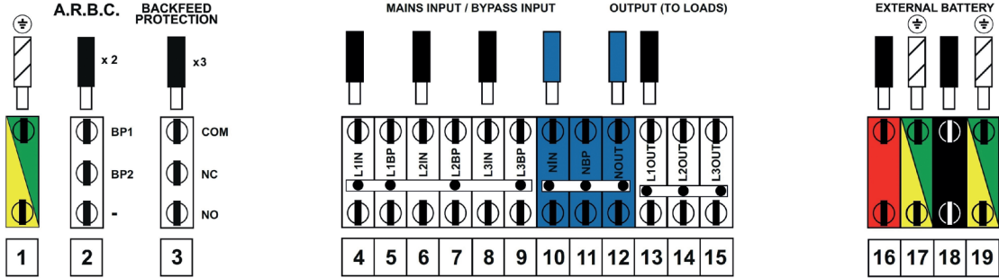
Trimod MCS 10 - 15 - 20 con linea di ingresso bypass in comune
