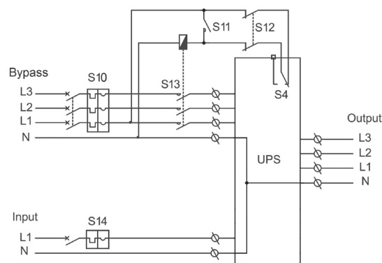
Configurazione Monofase/Trifase (disponibile solo per ingresso MONOFASE e uscita TRE FASI INDIPENDENTI)
