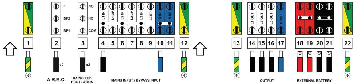
Trimod MCS 30 (linea di ingresso bypass disabilitata)
