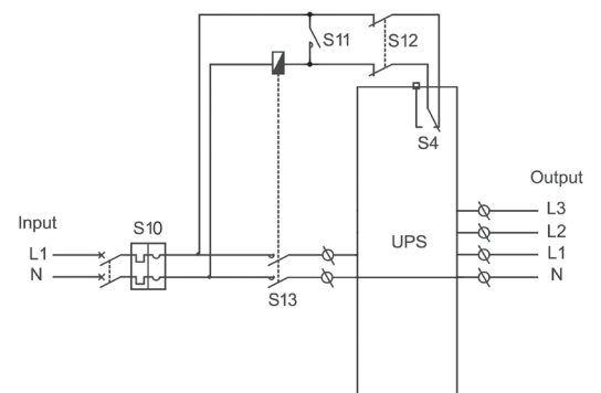
Configurazione Monofase/Trifase
