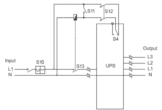
Configurazione Monofase/Trifase
