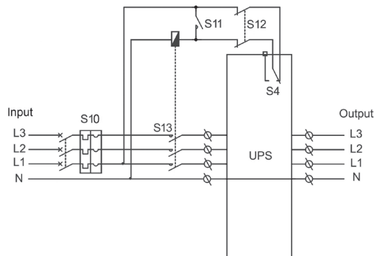
Configurazione Trifase/Trifase
