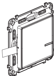
Bezdrôtový spínač
