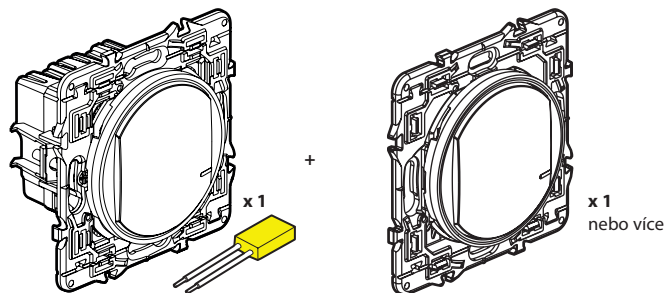
Spínač (s možností stmívání) + kompenzátor (není součástí kitu)
