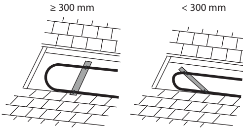
Pitää kaapelit erillään leveissä kouruissa Håller kablarna isär i breda rännor Keep cables apart in wide gutters Kaablivahe tagamiseks laiades rennides
