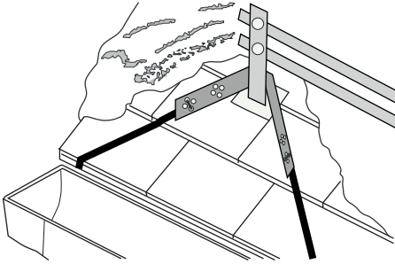
Kiinnitys lumiesteeseen Fäste i snöhinder Attaching to snow barrier Kinnitamine lumetökke külge
