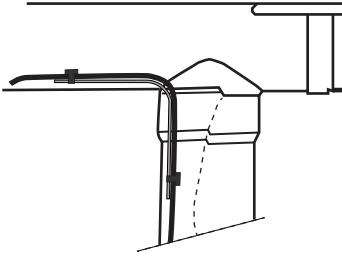
Räystäskouru, syöksytorvi Takränna, stupränna Gutter, drainpipe Vihmaveerenn, vihmaveetoru
