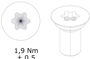
M5 x 10 (T25)
