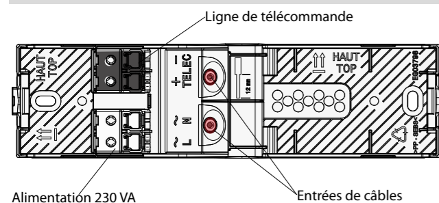
Alimentation 230 VA
