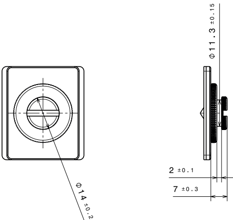
Button dimensions
