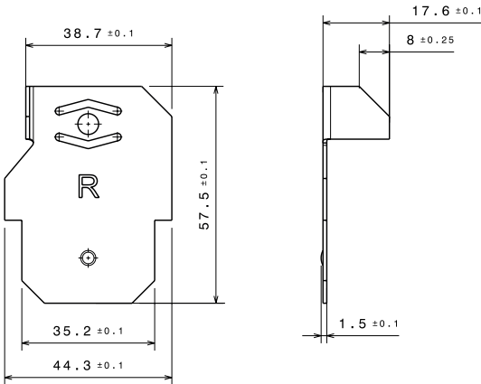
Dimensions de la patte de fixation NEXPAND
