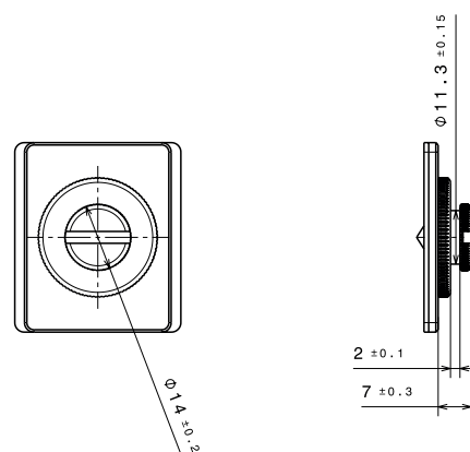
Dimensions du bouton
