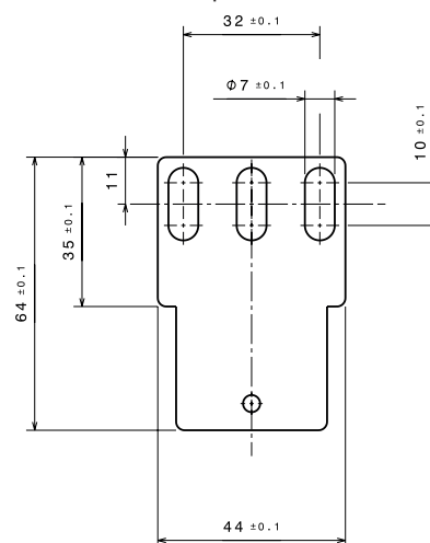
Dimensions de la patte de fixation standard
