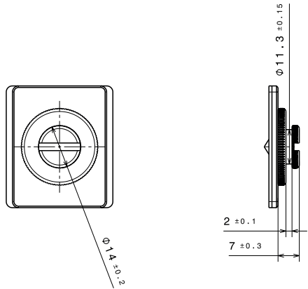
Dimensions du bouton
