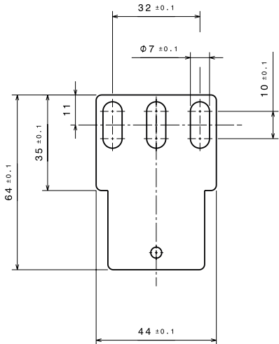
Dimensions de la patte de fixation standard
