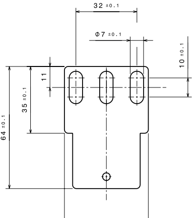
Dimensions de la patte de fixation standard
