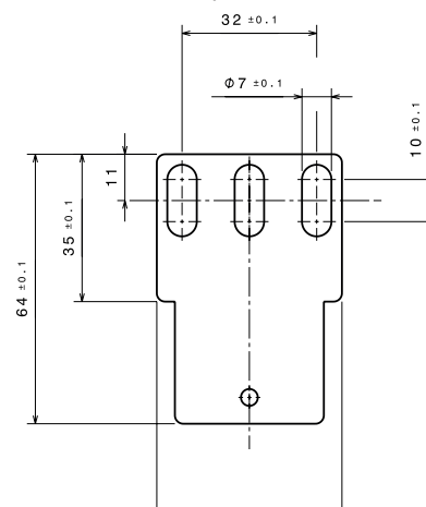
Dimensions de la patte de fixation standard
