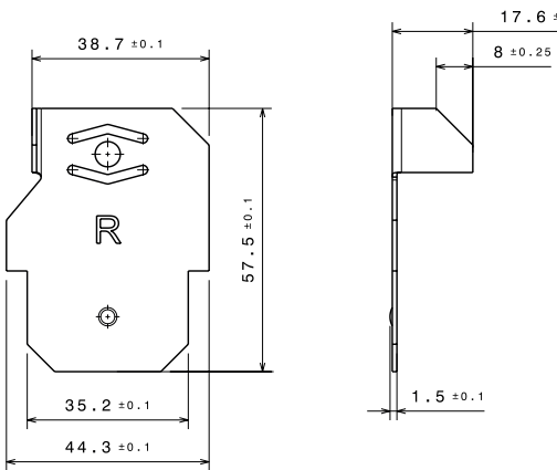
Dimensions de la patte de fixation NEXPAND
