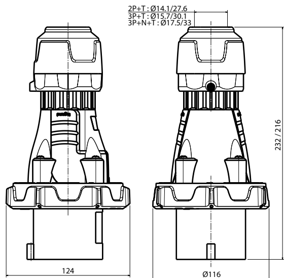
Prese mobili diritte 63 A
