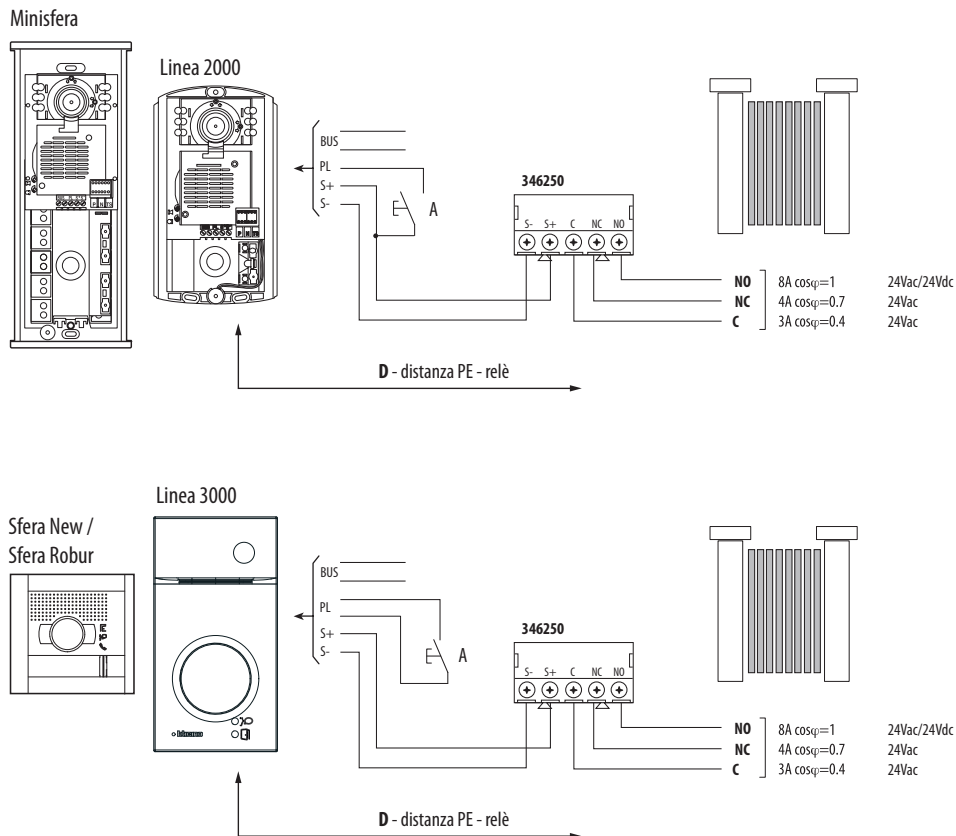
Distanza massima (D) in funzione del cavo utilizzato
