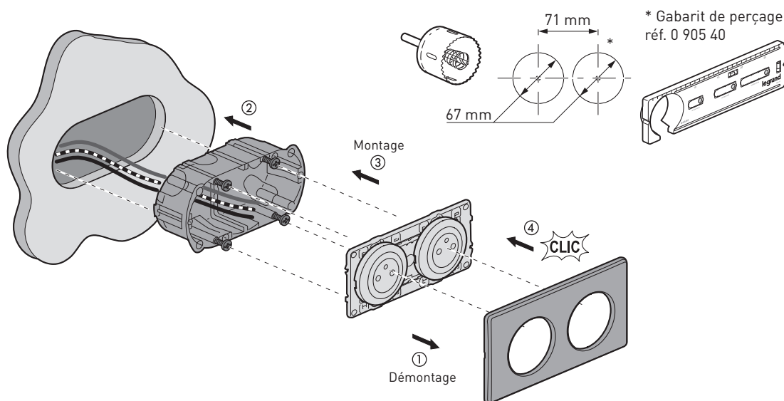
Connexion possible à gauche ou à droite
