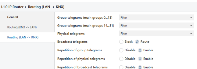
Fig. 5.3 Parameter window “Routing(LAN->KNX)”
