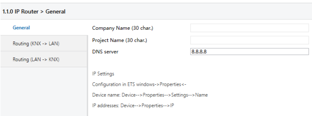
Fig 5.1.1 "General" parameter window
