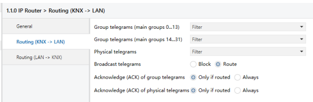
Fig. 5.2 Parameter window “Routing(KNX->LAN)”
