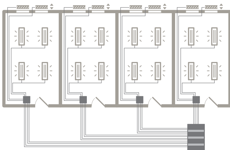
INSTALLATION CENTRALISÉE
