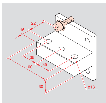
Accessoire de raccordement orientable pour DMX 3 débrochables tailles 4000 et 6300
