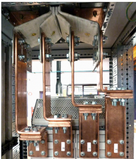
Kit de liaison entre DMX 3 taille 2500 débrochable et une arrivée SCP
