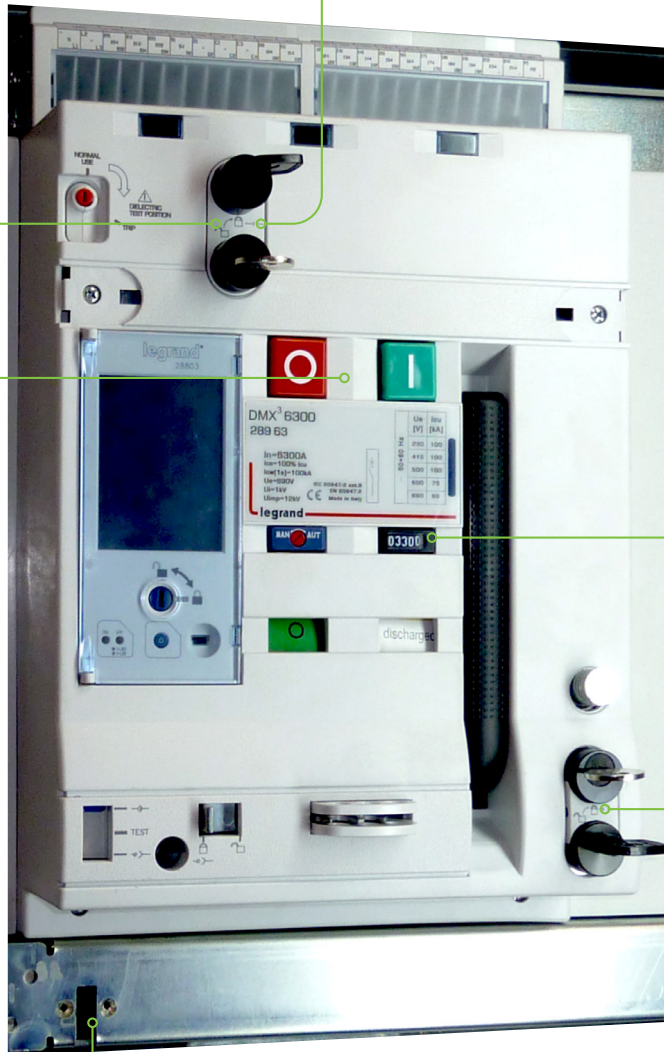
Cadenassage en position ouvert
