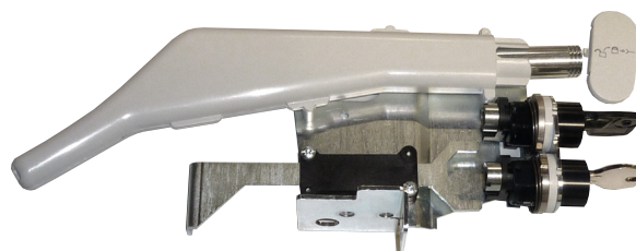
Accessoire de verrouillage réf. 0 288 32/33 équipé de deux barillets de types différents
