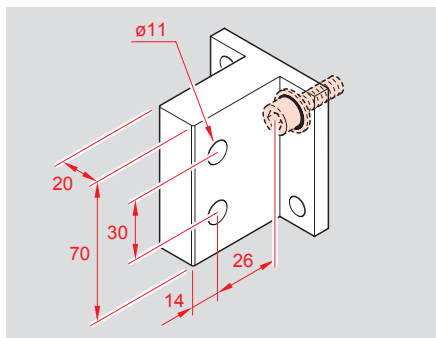
Accessoire de raccordement vertical pour DMX 3 fixes taille 2500
