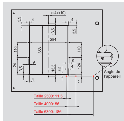
Plan de perçage du plastron pour un DMX 3 version fixe
