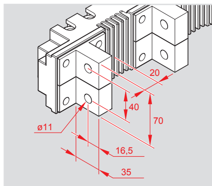
Accessoire de raccordement vertical pour DMX 3 fixes taille 2500
