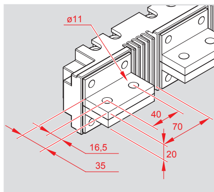
Épanouisseurs pour DMX 3 fixes taille 2500
