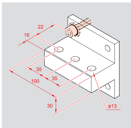
Accessoire de raccordement orientable pour DMX 3 fixes tailles 4000 et 6300
