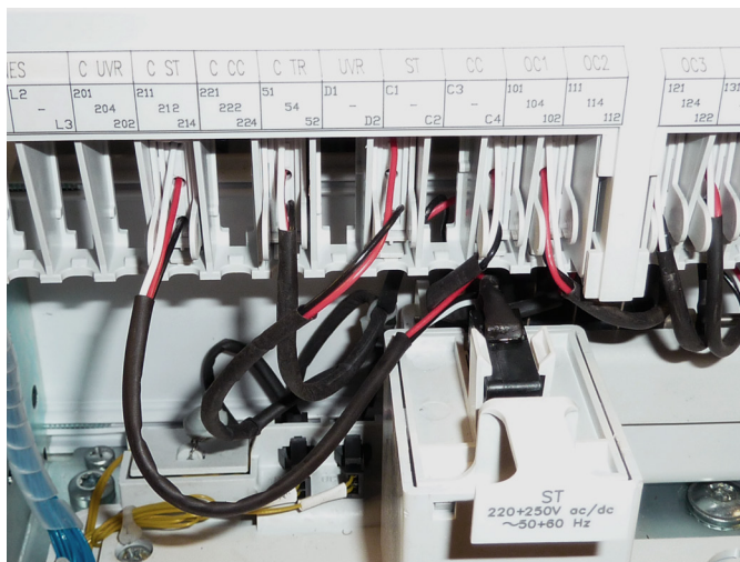
Le contact de signalisation se monte sur le dessus de la bobine ou des déclencheurs
