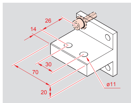
Accessoire de raccordement horizontal pour DMX 3 débrochable taille 2500
