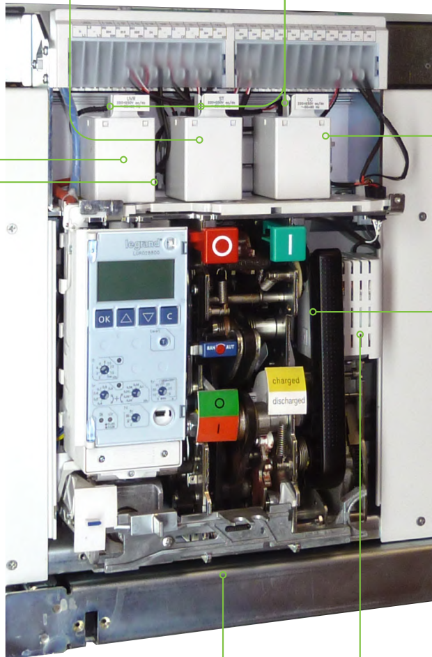
Déclencheur à émission de courant
