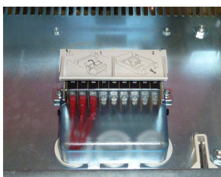
Le capot isolant assure la protection des bornes
