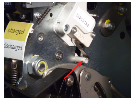
Ergot du contact SC
