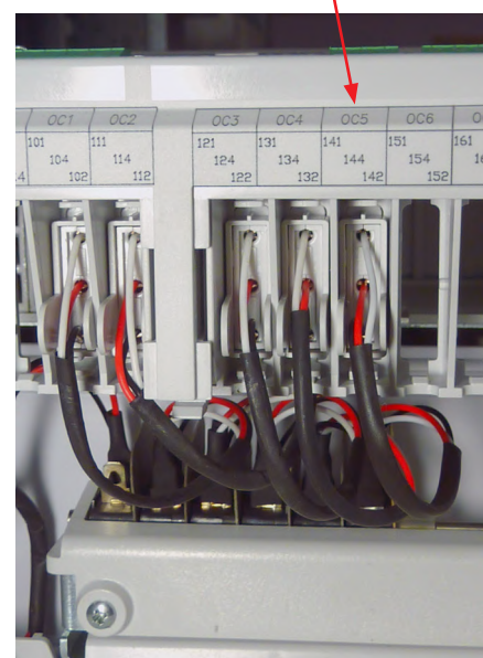
Quatre contacts auxiliaires pré-installés et un contact auxiliaire optionnel
