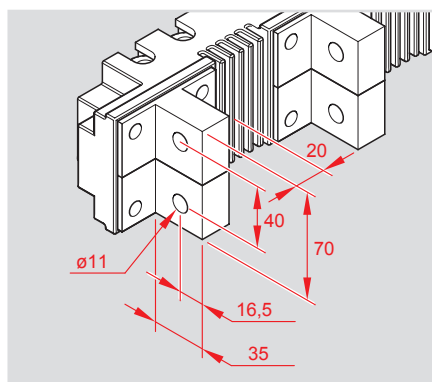
Accessoire de raccordement vertical pour DMX 3 fixes taille 2500
