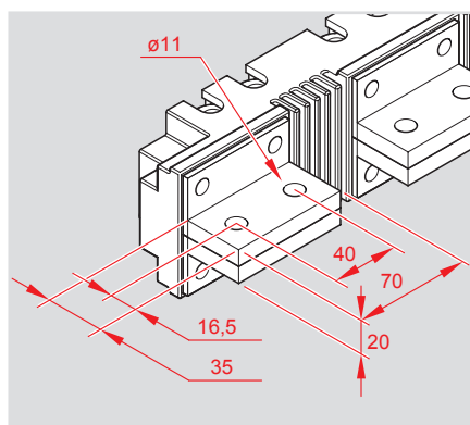
Épanouisseurs pour DMX 3 fixes taille 2500
