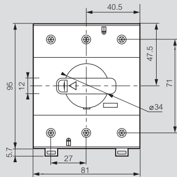
Frame 2, 3-pole Cat.Nos 4 240 03/04/05
