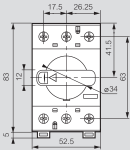
Frame 1, 3-pole Cat.Nos 4 240 00/01/02
