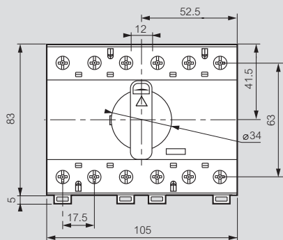
Frame 1, 3-pole, Cat.Nos 4 241 00/01/02
