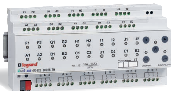
Contrôleur modulaire ON/OFF multi-application, 20 sorties
