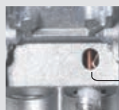
Als de kern van de coax hier zichtbaar is dan is er een goed contact verzekerd
