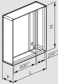
Vloerkasten met interne kabelmantel
