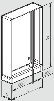
Vloerkasten met interne kabelmantel
