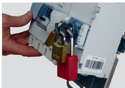
Insérer les cadenas.
