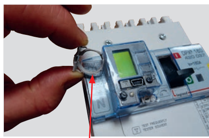
Support de batterie
