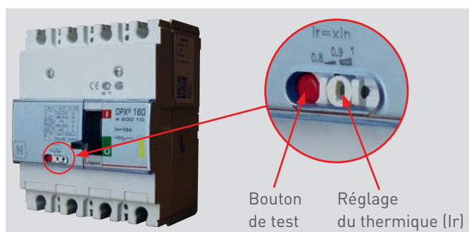
DPX 3 160 magnétothermique.
