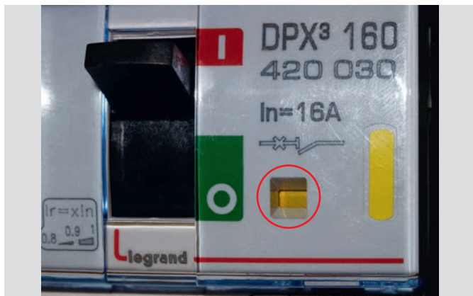
Déclenché sur défaut différentiel.
