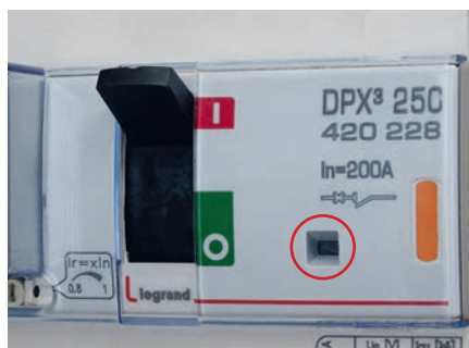
Fermé (ON)
