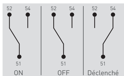
Sortie latérale.
