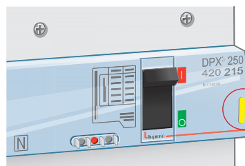
DPX 3 250 Montage sur rail ou sur platine
