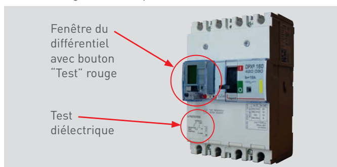
DPX 3 160 magnétothermique avec différentiel.
