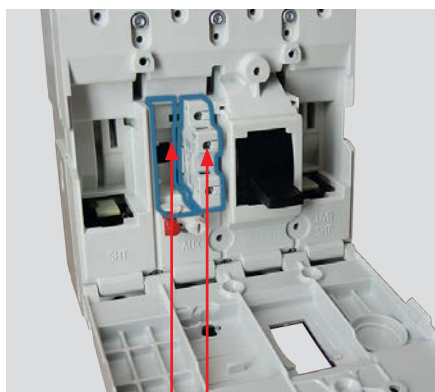
Sortie sur le dessus.
