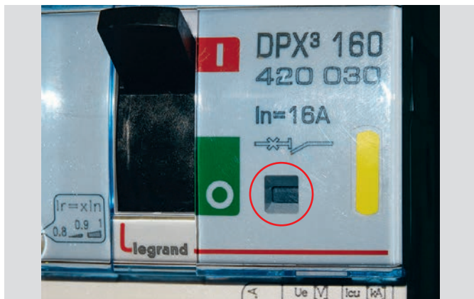
Fermé (0N).
