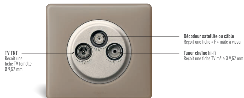
PRISE TV-FM-SAT CÉLIANE | GRÈS
