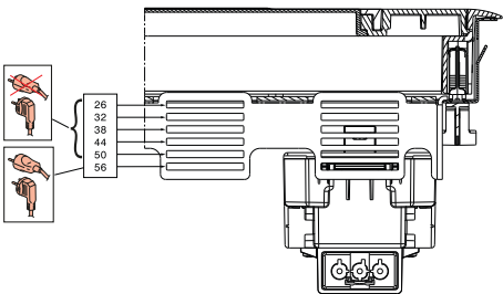
Dimensions (mm) des différentes positions du module
