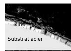
Coupe GC x 200 après pliage puis test à 550 h BS
