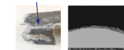
Tôle ZnMg pliée ZnMg x 100 après déformation puis test 2000 h BS :
