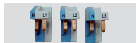
JEU DE 3 MODULES DE CONNEXION 1P+N RÉF. 4 052 51
