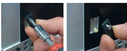
Avant montage du DPX 3 , retirer la plaquette située à l'arrière du produit pour libérer la tige qui permettra de déclencher le disjoncteur dès lors que le tiroir (partie mobile) ne sera plus en contact avec la base (partie fixe).
