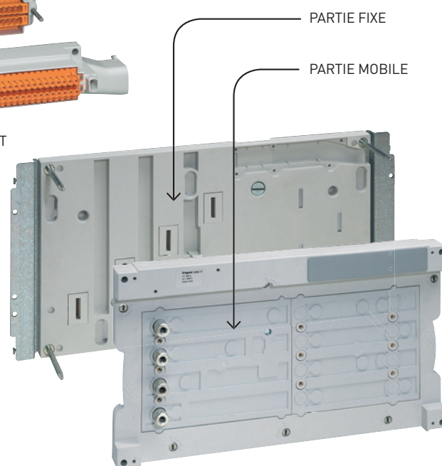
BASE IS 223 POUR DPX 3 630
