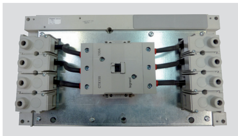
EXEMPLE D'UN CONTACTEUR POUR DÉPART MOTEUR MONTÉ SUR BASE UNIVERSELLE 233
