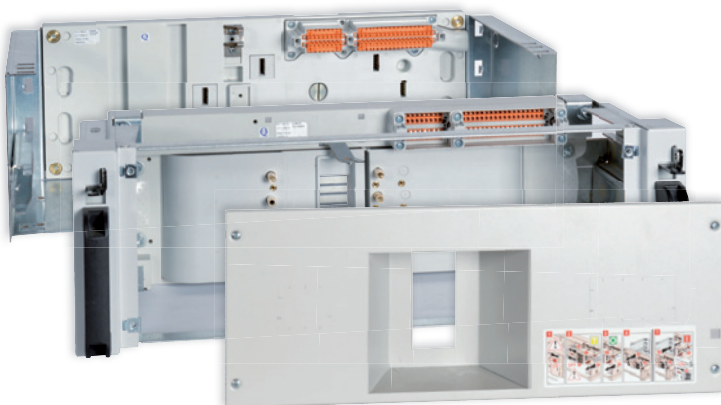
Base VX 3 IS 333 pour DPX 3 250 et plastron dédié (à commander séparément)
