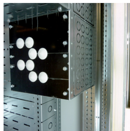
L'utilisation des caissons de cloisonnement pour les raccordements aval en IS 233/333 permet d'obtenir le niveau de forme 4b.
