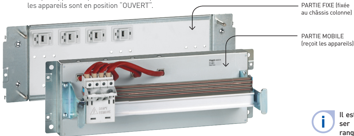
RÉPARTITEUR DE RANGÉE HX 3 IS 125 A
