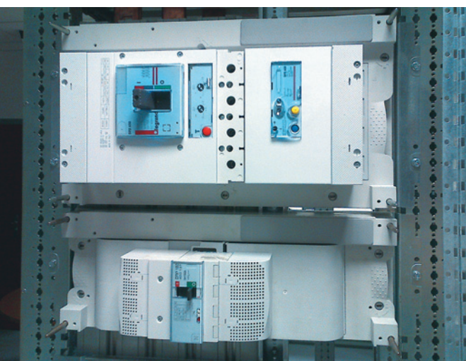
Les disjoncteurs DPX 3 se montent en position horizontale sur les bases.
