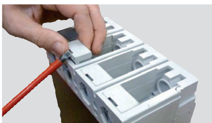
Retirer les huit entretoises plastique des bornes amont et aval de l'appareil.
