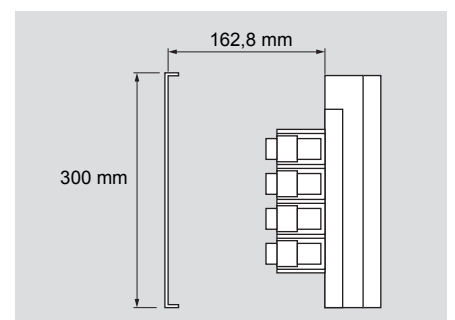
Volume disponible sous plastron.
