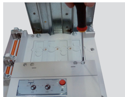
Les fixer à l'aide des vis fournies (deux par cache-bornes).
