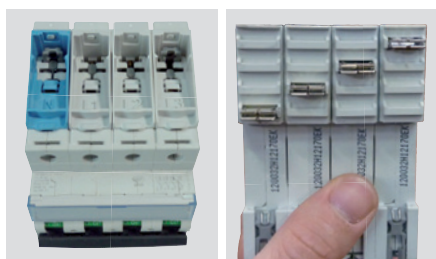
DISJONCTEUR 4 PÔLES ÉQUIPÉ DE SES 4 MODULES DE CONNEXION
