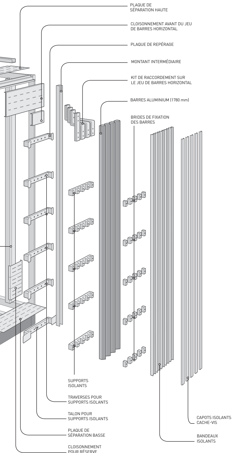
Les cloisons pour réserve garantissent le niveau de forme 3b, requis pour les IS 223, 233 et 333.
