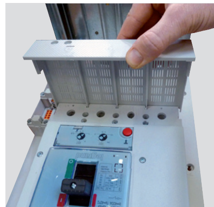
Insérer les cache-bornes sur l'appareil.
