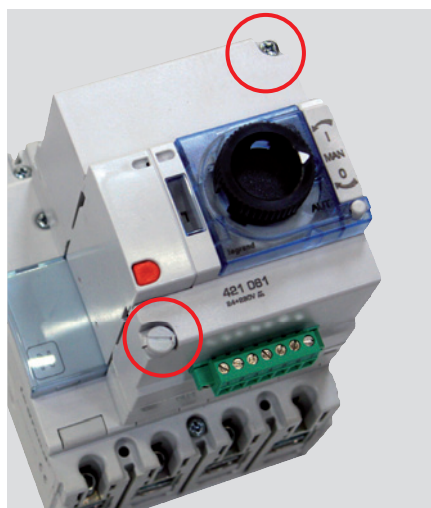
Fixer le moteur sur son embase en utilisant les deux vis en diagonale.
