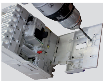
Percer le capot du disjoncteur comme indiqué dans la notice.
