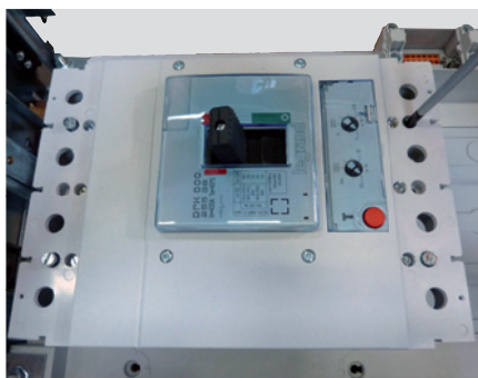
Le fixer à l'aide des quatre vis fournies avec le disjoncteur (couple de serrage : 1 Nm).
