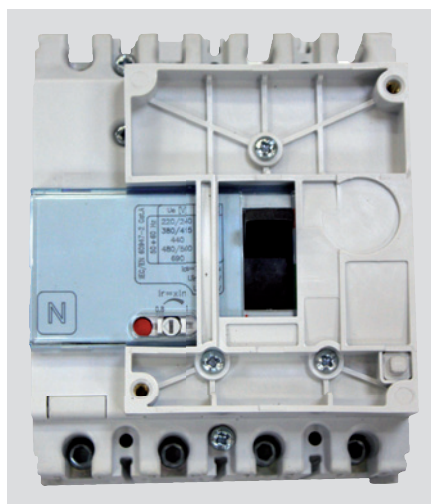
Fixer l'embase de la commande motorisée à travers les perçages précédemment réalisés.
